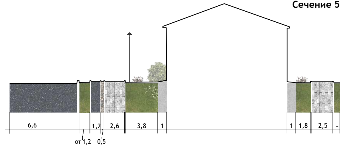
Сечение 5
